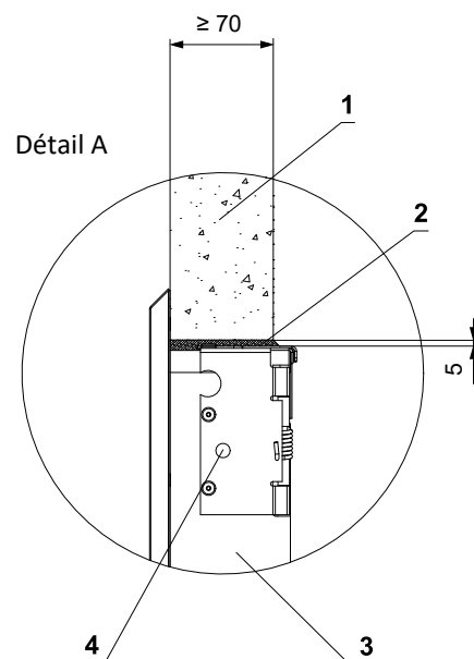
Détail de la connexion du volet avec le conduit
