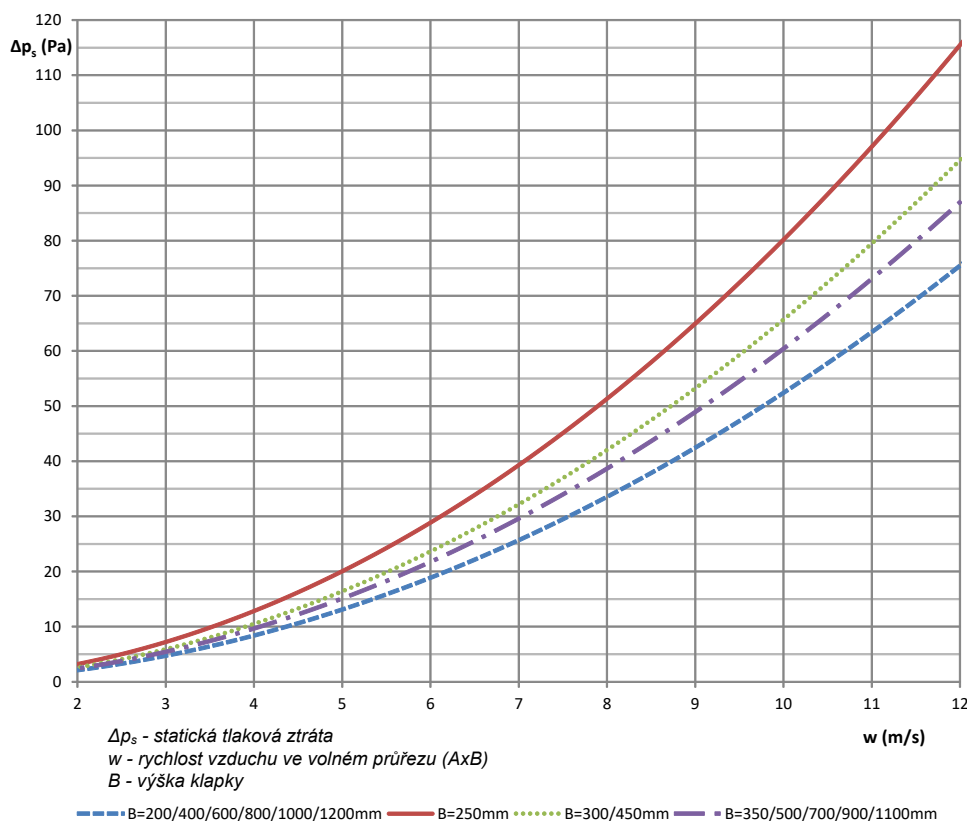
Diagram 1 Tlaková ztráta klapky byla stanovena na hustotu vzduchu 1,2 kg/m 3
