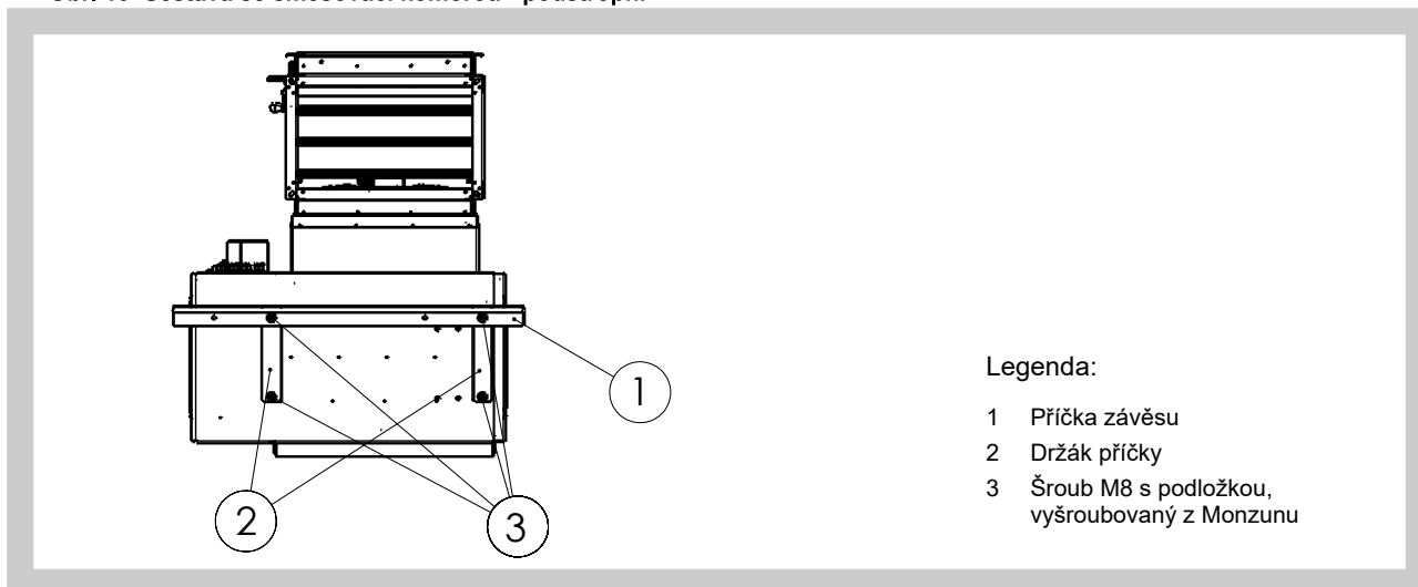
Obr. 10 Sestava se směšovací komorou - podstropní
