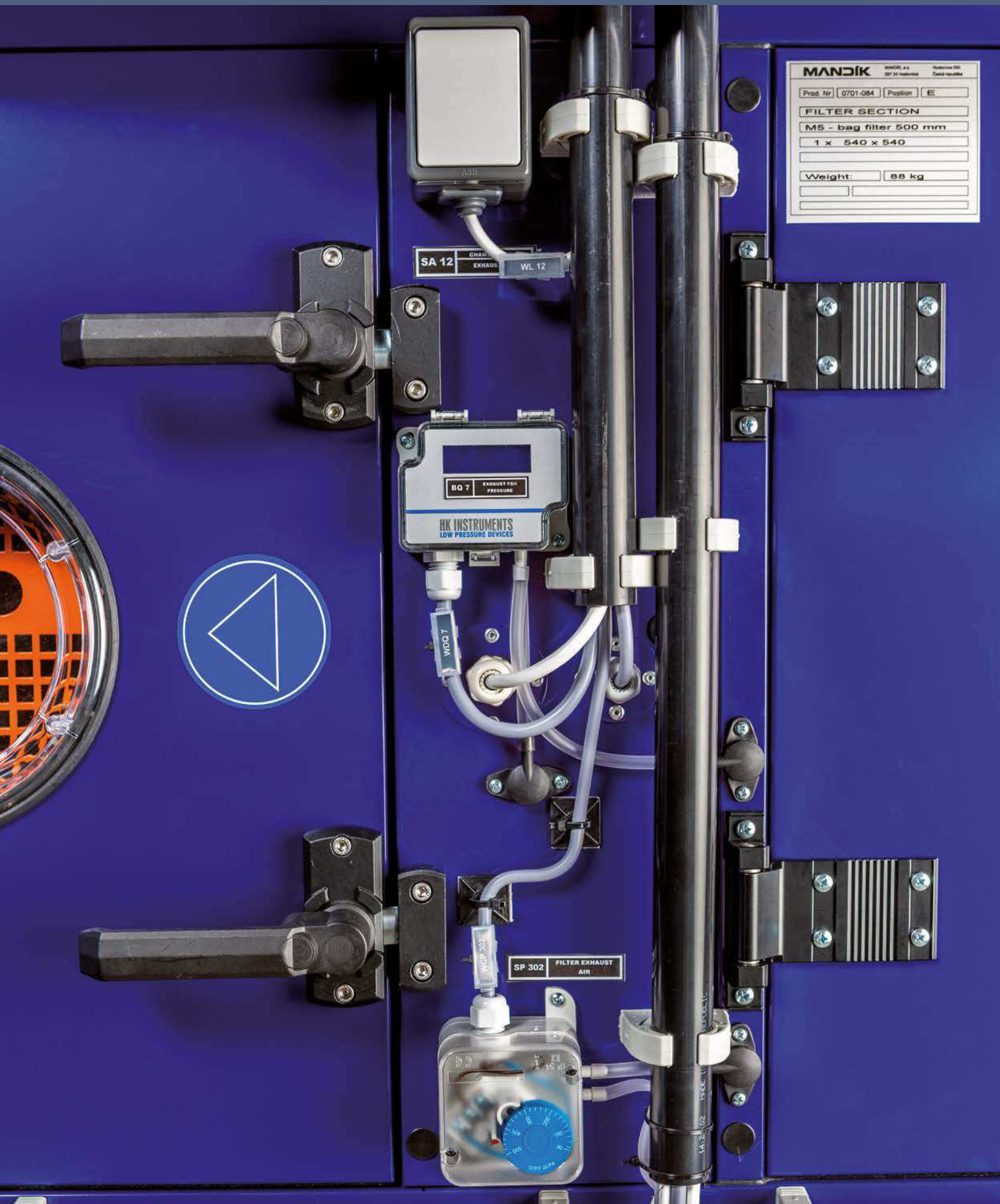
» M3.15 detail umístění kabeláže a vypínačů osvětlení
